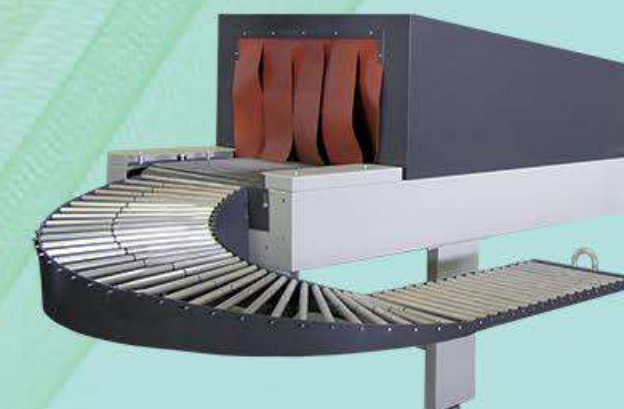
TUNNEL TTN CON RULLIERA IN CURVA
